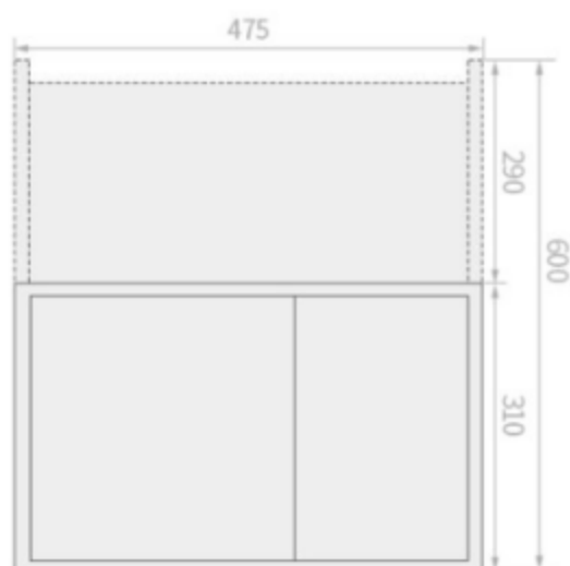
●正视图(展开)
