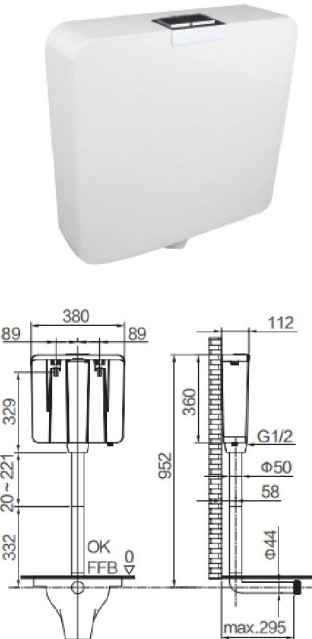
RA-B692挂壁水箱
