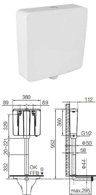
RA-B691挂壁水箱
