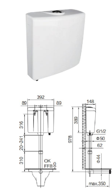
RA-B685挂壁水箱
