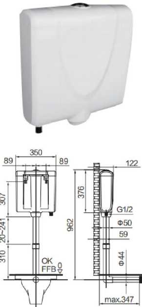
RA-B690挂壁水箱
