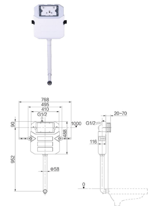
RA-K130-D02系列隐藏水箱，配蹲厕
