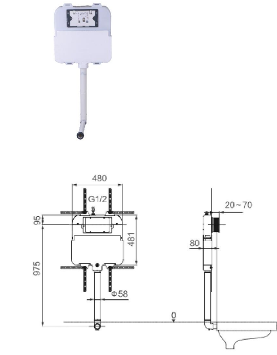
RA-K301-D02系列隐藏水箱，配蹲厕
