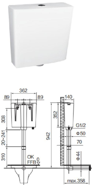
RA-B687挂壁水箱
