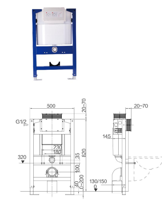
RA-K210-A01系类隐藏式水箱
