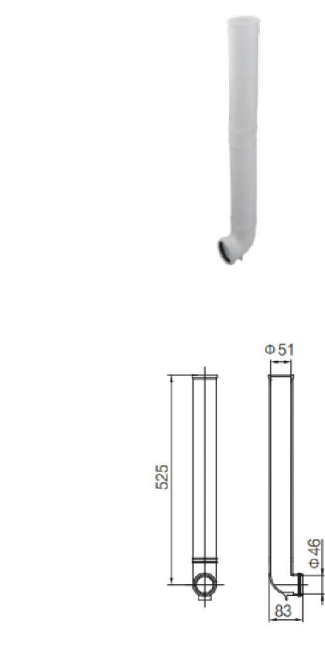
RA-9045加长冲刷弯管
