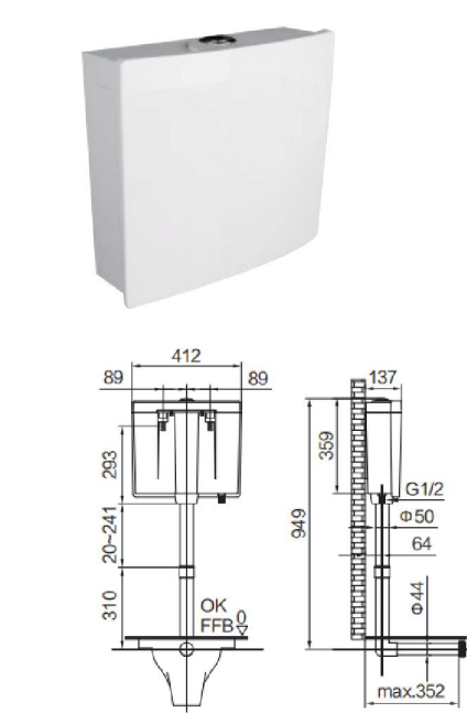
RA-B690挂壁水箱
