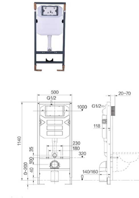
RA-K-130A02系列隐藏水箱 (配8016机架) 高度1140MM
