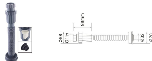
浴室柜、面盆下水管
