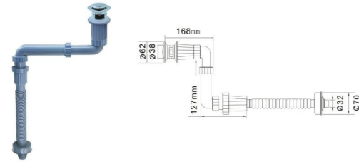
浴室柜、面盆下水器
